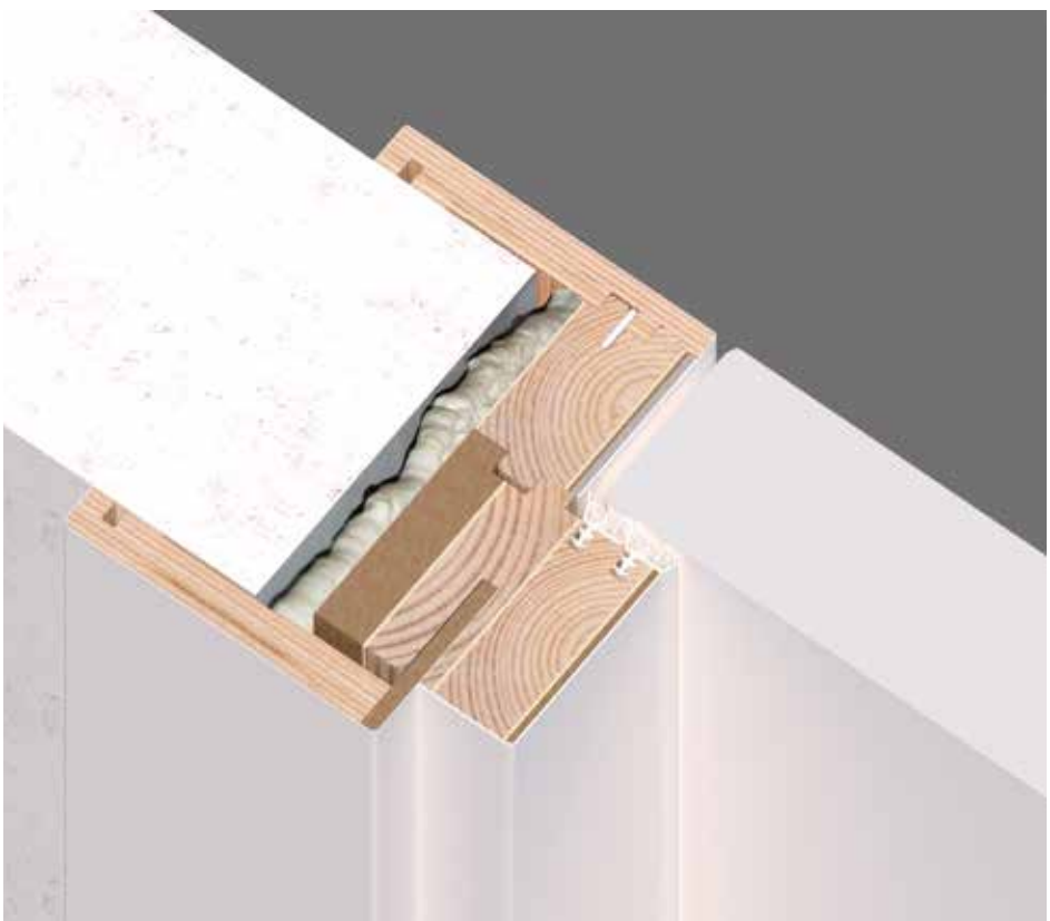
HTB-S7 / push side 41dB - EI 1 30 / EI 2 45
